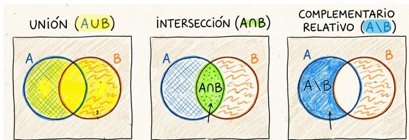
Figura 1. Representación «ingenua» de la unión, la intersección y el complementario relativo.
