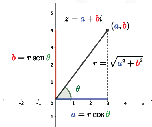
Figura 7. Representación gráfica de un número complejo
