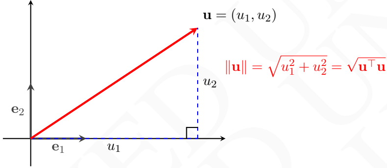
Figura 14. Interpretación geométrica del módulo de un vector mediante el teorema de Pitágoras en \mathbb{R}^2 .
