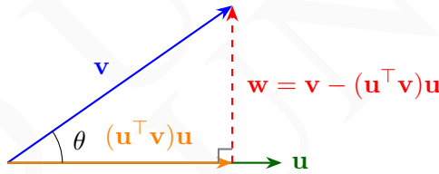
Figura 16. Los vectores \mathbf{u} y \mathbf{v} son aquí unitarios.
