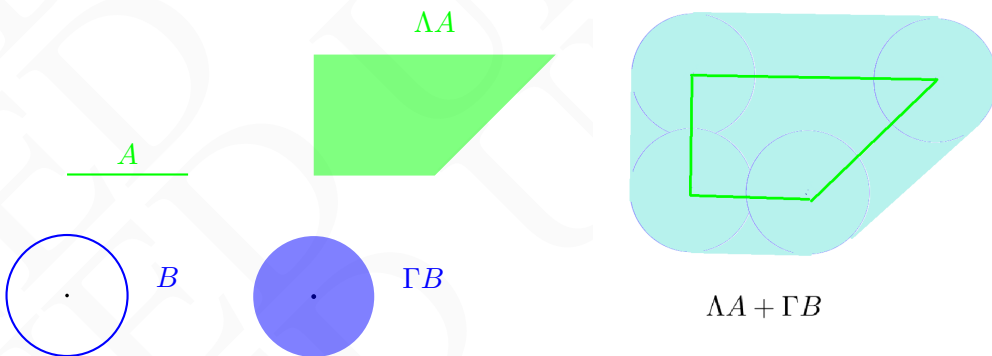
Figura 11. Dibujos correspondientes al ejemplo 47.
