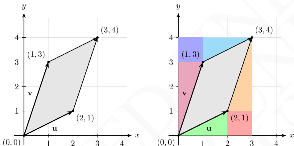
Figura 17. Paralelogramo generado por las columnas de la matriz A .
