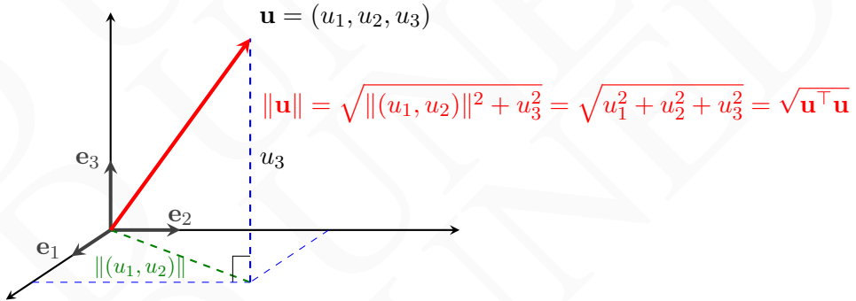
Figura 15. Interpretación geométrica del módulo de un vector mediante el teorema de Pitágoras en \mathbb{R}^3 .
