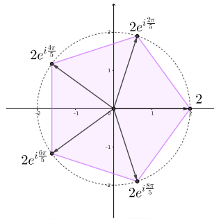
Figura 9. Raíces de un número complejo
