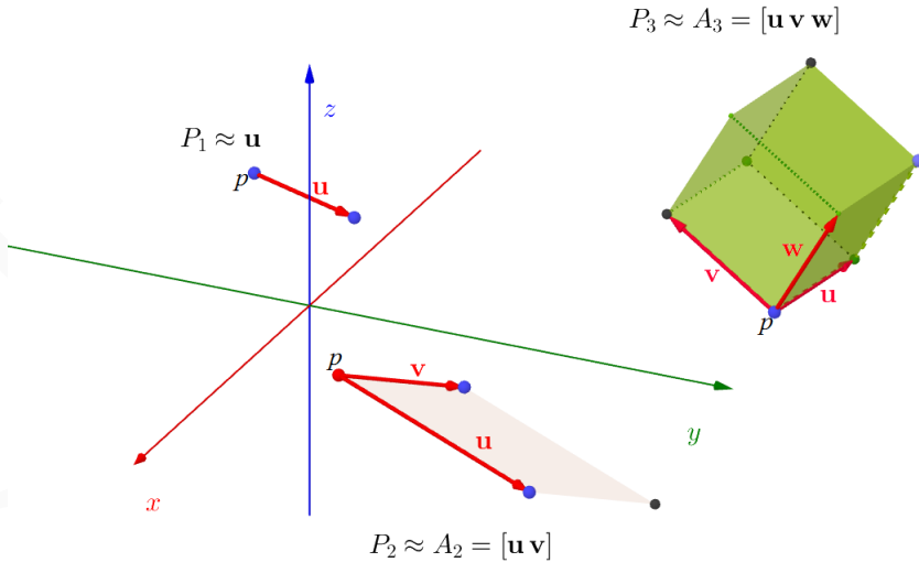
Figura 18. Al segmento P_1 se le asigna un elemento de \mathbb{R}^n \equiv \mathbb{R}^{n \times 1} (vector); al paralelogramo P_2 , una matriz de \mathbb{R}^{n \times 2} (par de vectores); al paralelepípedo P_3 , una matriz de \mathbb{R}^{n \times 3} (terna de vectores), etc.
