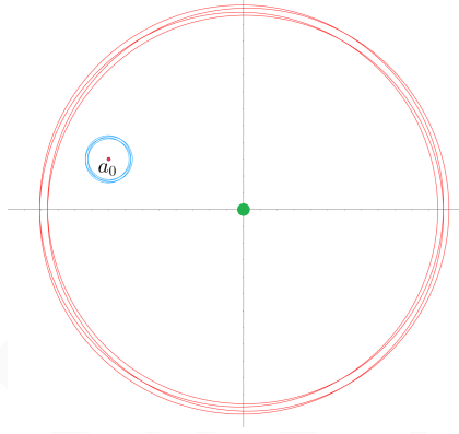
Figura 10. En azul, la curva w(\theta) = P(re^{i\theta}) para r \approx 0 ; en rojo, para r \gg 0 .
