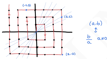
Figura 4. Una manera de enumerar los números racionales (saltándose repeticiones).
