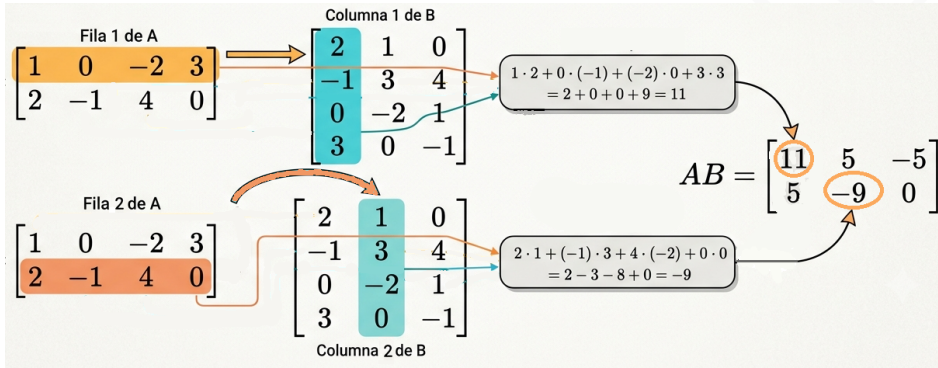
Figura 13. Producto de matrices del ejemplo 69.
