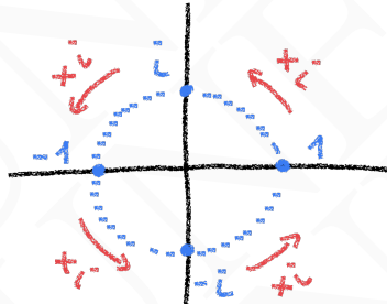
Figura 8. Interpretación geométrica de la multiplicación por la unidad imaginaria.
