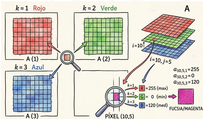
Figura 12. Una imagen RGB como conjunto de números indexado por tres índices.
